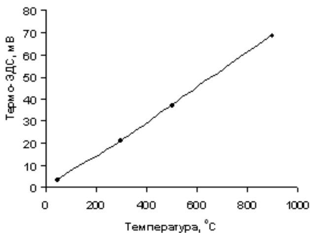
Рисунок 1 – График зависимости термо-ЭДС от температуры
