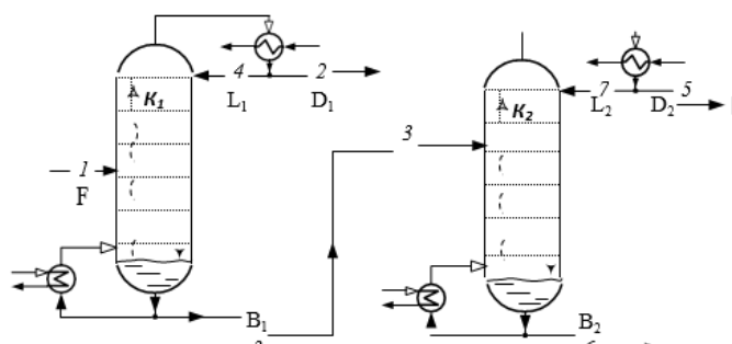
Рис. 2.1. 1 – сырье (хлорметил-изобутиленовая фракция); 2, 5 – хлорметилловая фракция; 3 – изобутиленовая фракция с примесью хлорметила; 4, 7 – флегма; 6 – изобутиленовая фракция
